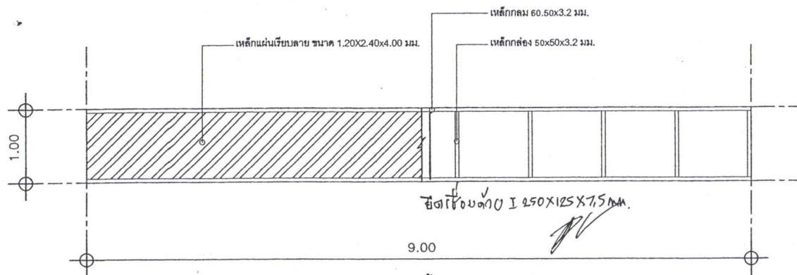
แปลนพื้น SCALE 1 : 50
