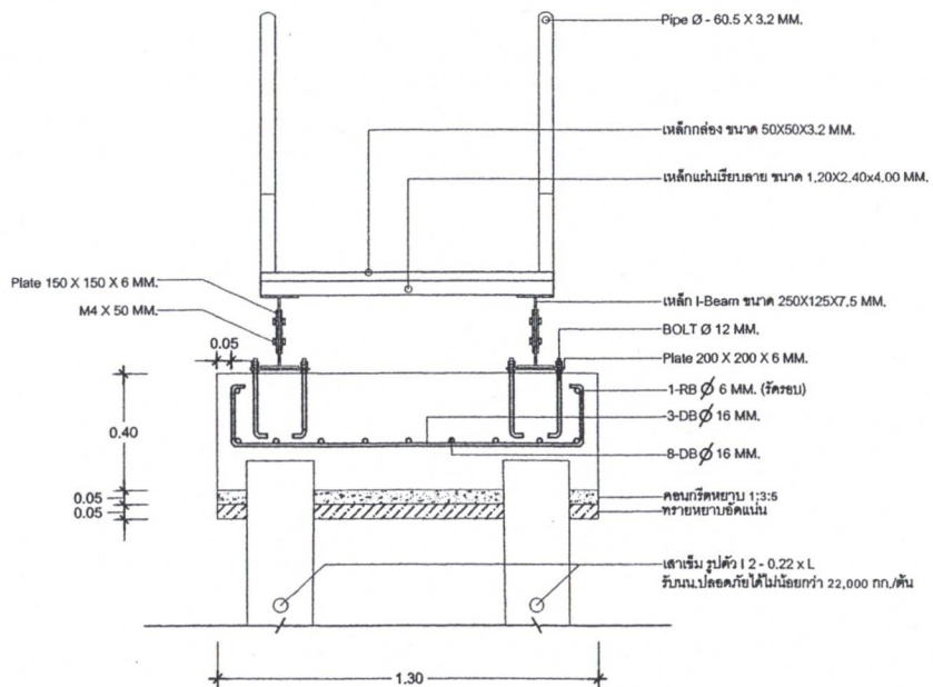
แปลนฐานราก F1 SCALE 1: 20
