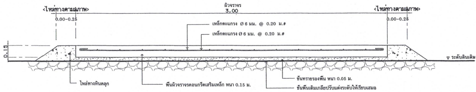
แบบแปลนรูปตัดถนนผิวจราจรคอนกรีตเสริมเหล็ก 1 : 20
