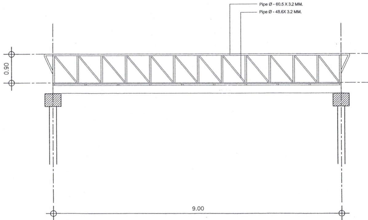
แปลนรูปด้านข้าง SCALE 1 : 50
