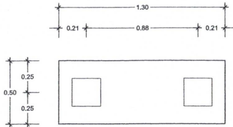
แปลนฐานราก F1 SCALE 1: 20
