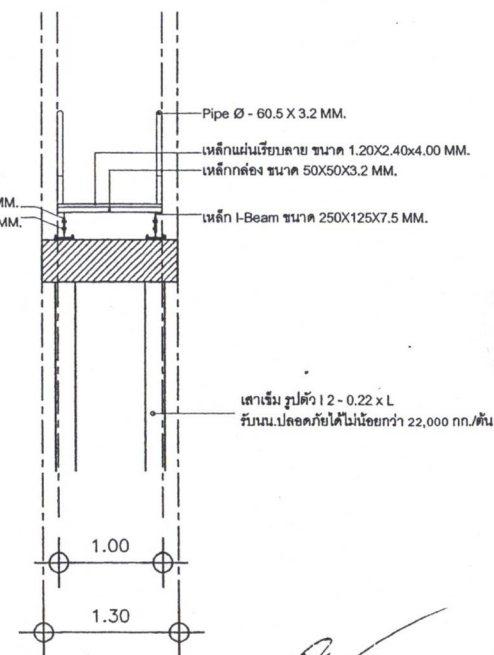
แปลนรูปด้านหน้า SCALE 1 : 50
