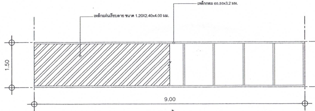
แปลนพื้น SCALE 1 : 50
