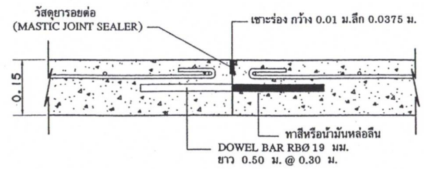
แบบแปลนขยายรอยต่อ CONSTRUCTION JOINT 1 : 10
